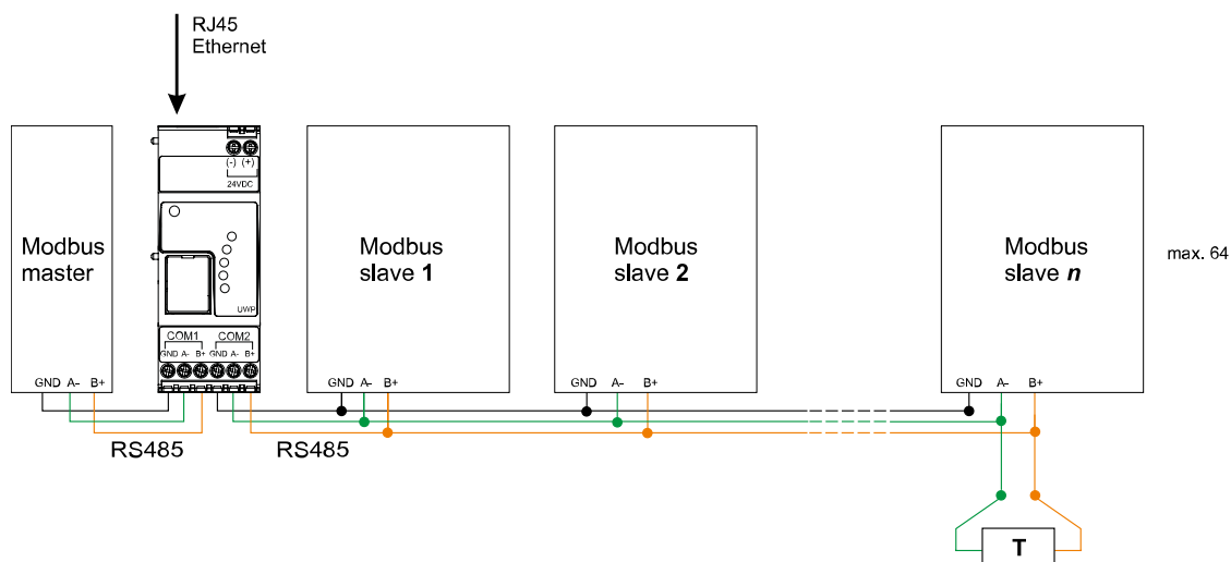
Fig. 1 Collegamento Modbus RTU Master COM 1, master COM 2
