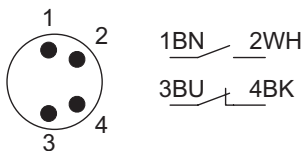
1NC + 1NA, versión conector
