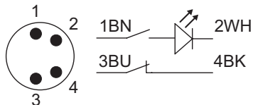
1NC + 1NA, versión conector con LED
