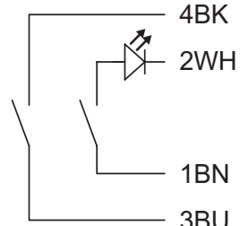
2NA, versión cable con LED
