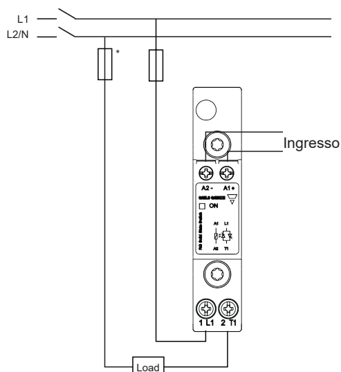
Variante senza protezione per Sovratemperatura
