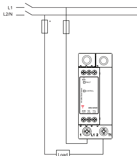
Variante con protezione per Sovratemperatura
