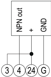
Fig. 13 Ingresso a impulsi NPN (codice prodotto: 2TIW)
