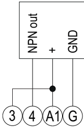
Fig. 15 Ingresso a impulsi NPN (codice prodotto: 2TCW)
