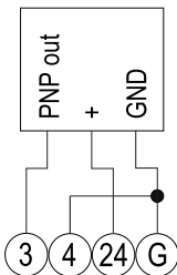
Fig. 14 Ingresso a impulsi PNP (codice prodotto: 2TIW)
