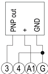
Fig. 16 Ingresso a impulsi PNP (codice prodotto: 2TCW)
