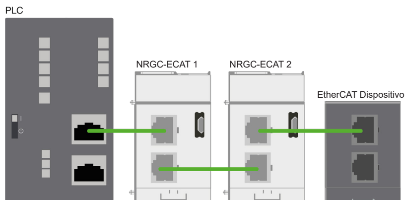
Fig. 3 Esempio di una configurazione in linea di NRGC-ECAT con altri dispositivi e controllore in EtherCAT
