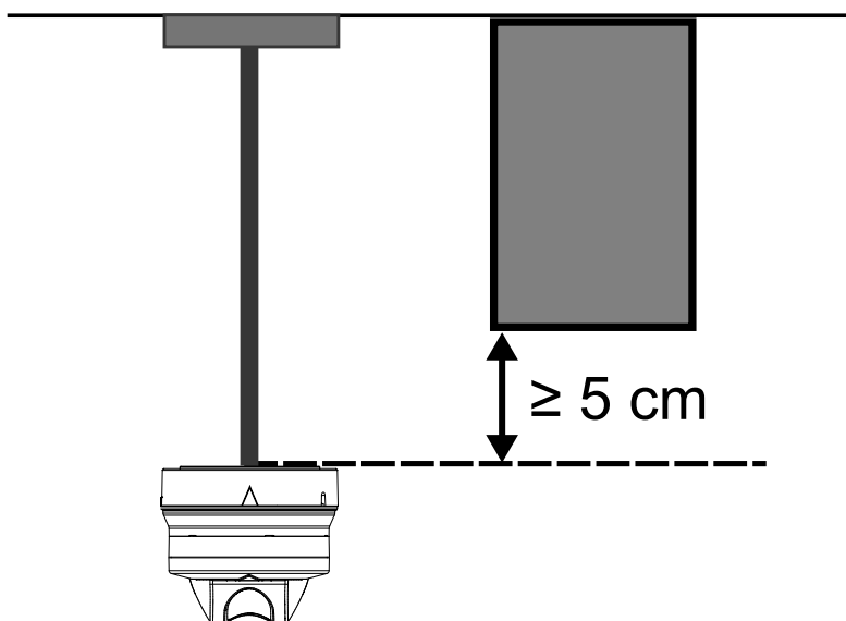
Fig. 5 La base del sensore deve essere almeno 5 cm sotto l'ostacolo
