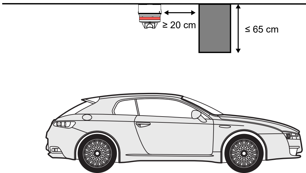
Fig. 4 Gli ostacoli riducono la capacità di rilevamento del sensore
