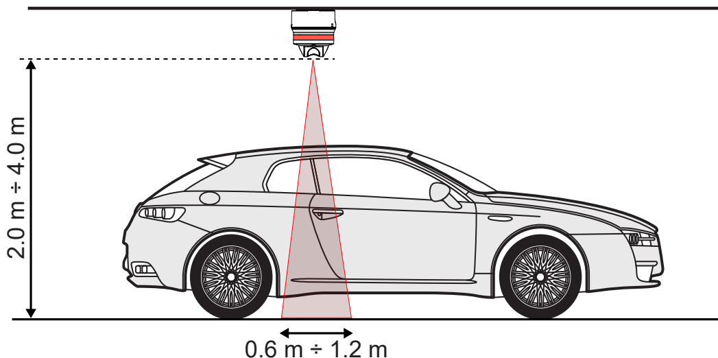
Fig. 3 Altezza e distanza del sensore
