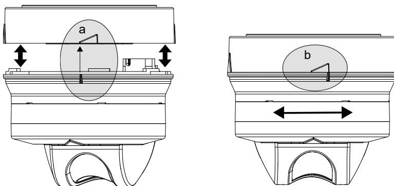
Fig. 7 Montaggio / Smontaggio
