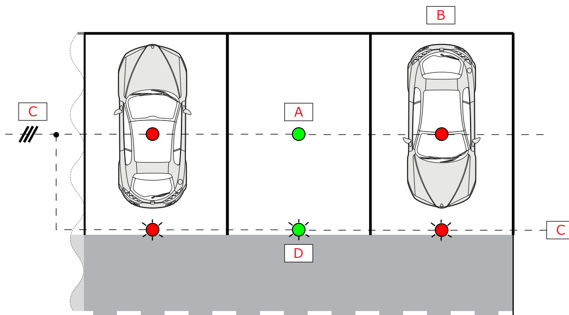
Fig. 9 Installazione del sensore - SBPSUSL associati agli indicatori SBPILED
