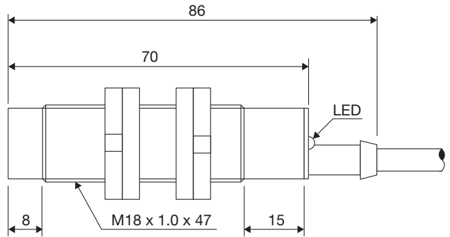
Fig. 7 Cavo CA18CAN...A2IO
