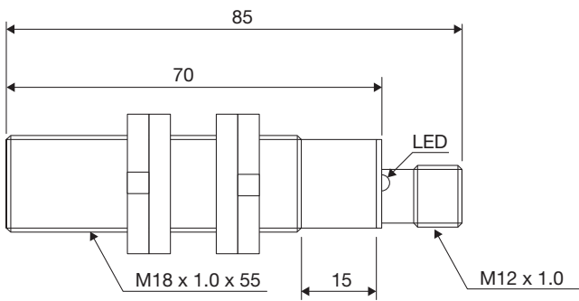
Fig. 8 Connettore CA18CAF...M1IO
