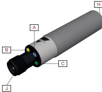
Fig. 2 CA18 Connettore
