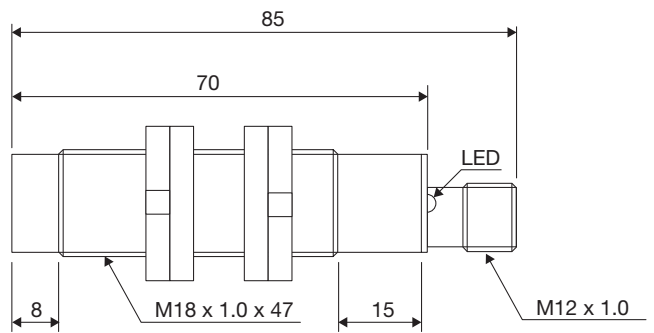
Fig. 9 Connettore CA18CAN...M1IO
