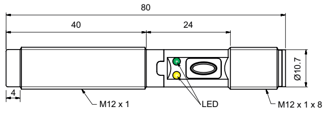
Fig. 7 Connettore
