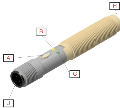
Fig. 2 Connettore
