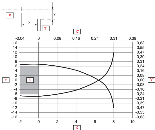
Fig. 4 A filo
