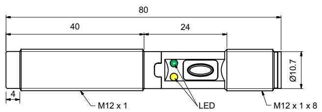
Fig. 9 Connettore CA18EAN...M1IO
