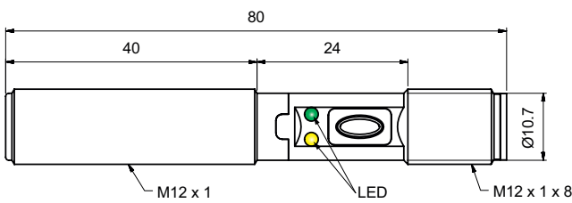
Fig. 8 Connettore CA18EAF...M1IO
