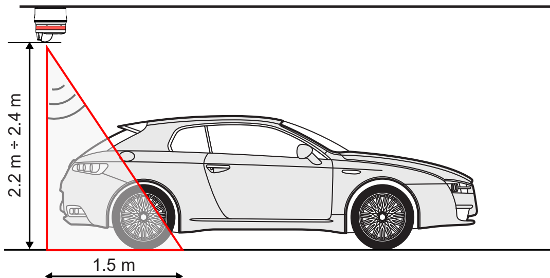
Fig. 1 Hauteur d'installation et distance de détection du capteur
