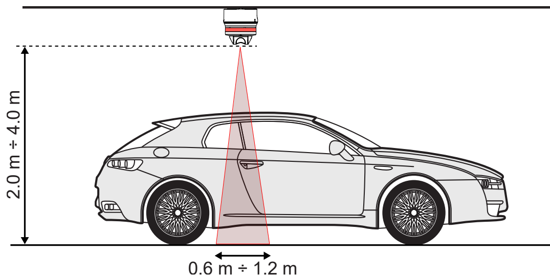
Fig. 2 Hauteur d'installation et distance de détection du capteur
