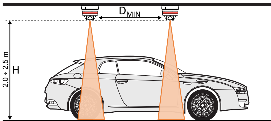
Fig. 3 Hauteur du capteur
