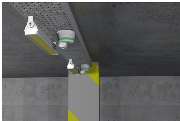
Mettre SBPBASEA avec le capteur devant la lampe DEL
