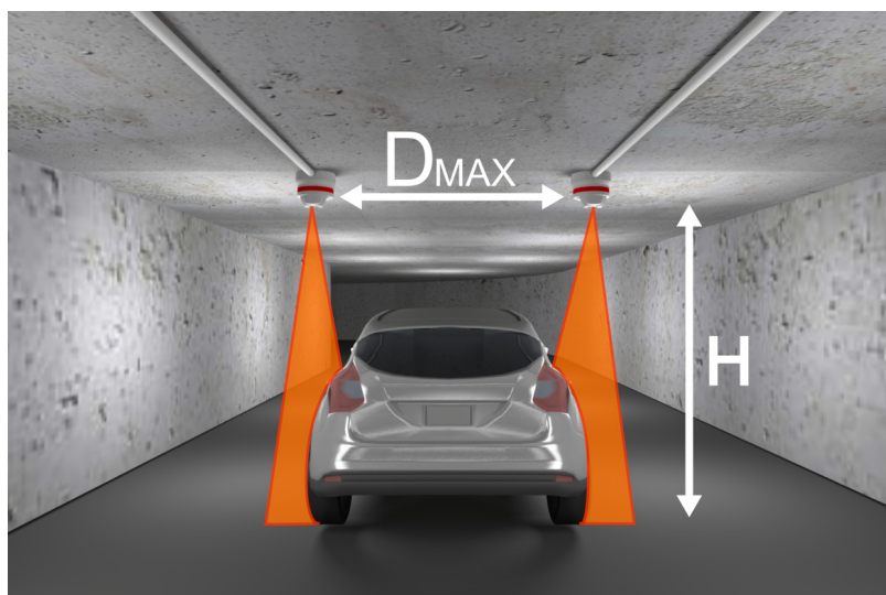
Fig. 4 Hauteur du capteur
