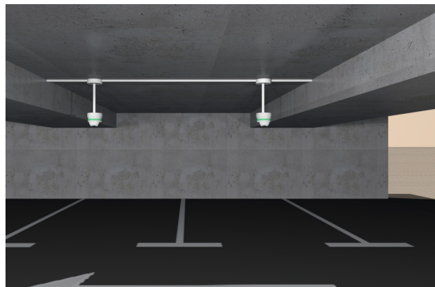
Mettre le SBPBASEA au minimum à 5 cm au-dessous des obstacles
