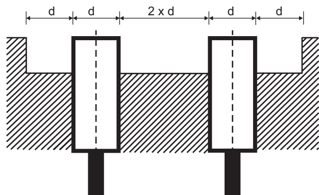
Fig. 13 Sensores no empotrados, cuando se instalan juntos en material detectable
