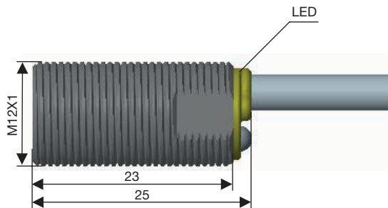
Fig. 6 Caja corta, para montaje empotrado, cable
