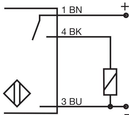
Fig. 4 PNP - Normalmente abierto
