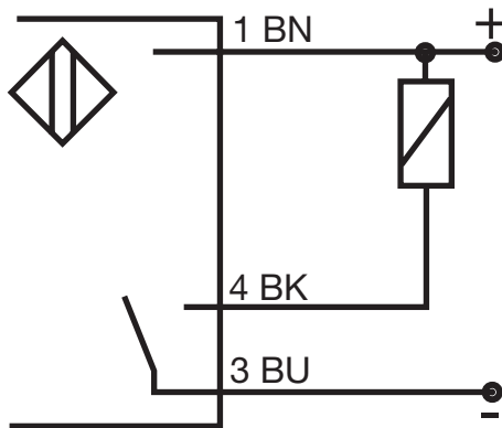
Fig. 2 NPN - Normalmente abierto
