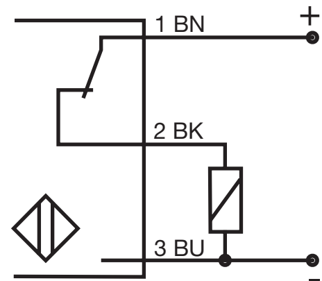
Fig. 5 PNP - Normalmente cerrado
