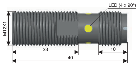
Fig. 8 Caja corta, para montaje empotrado, conector
