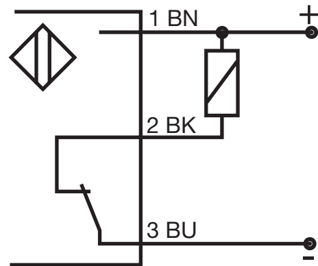
Fig. 3 NPN - Normalmente cerrado
