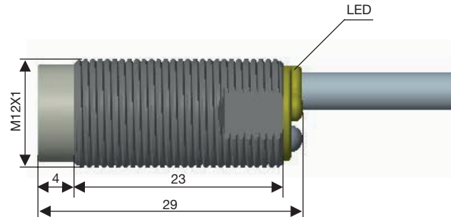
Fig. 7 Caja corta, para montaje no empotrado, cable
