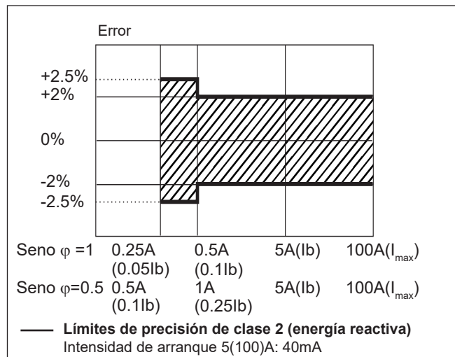
kvarh, precisión (lec.) dependiendo de la intensidad
