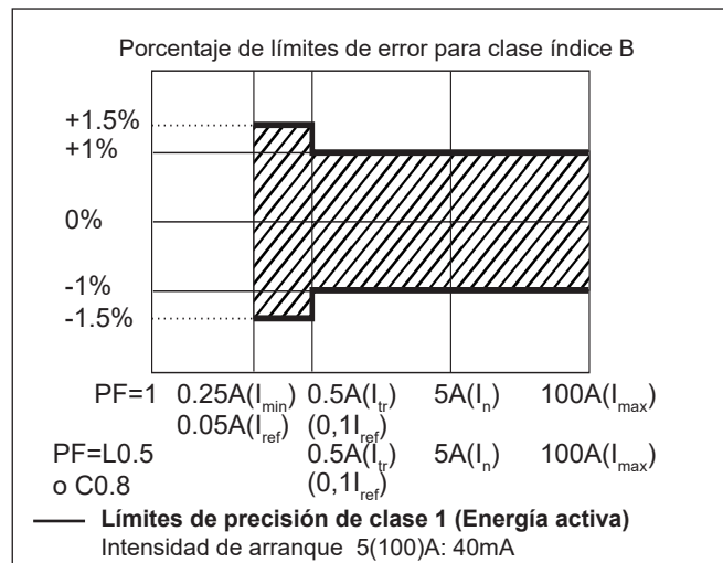
kWh, precisión (lec.) dependiendo de la intensidad
