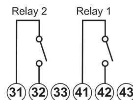
Fig. 27 Salidas de relé
