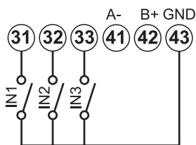
Fig. 28 Entradas digitales
