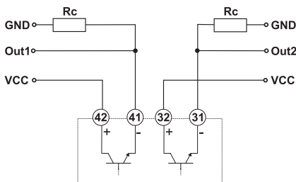
Fig. 26 Salidas estáticas, referencia VCC
