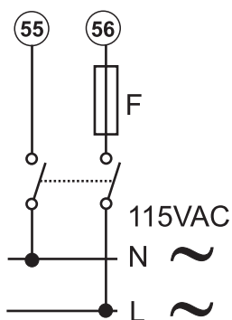
Fig. 23 Opción D. F = 250 V, 100 mA
