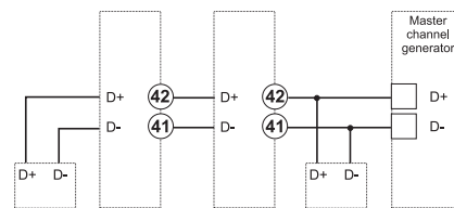
Fig. 30 Puerto Dupline
