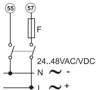
Fig. 24 Opción L. F = 250 V, 200 mA
