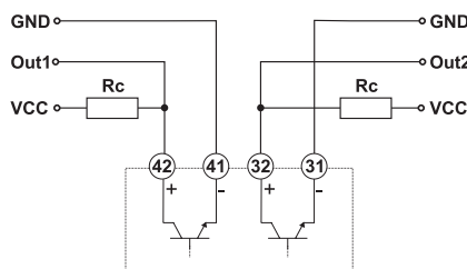
Fig. 25 Salidas estáticas, referencia GND (Tierra)
