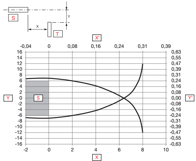
Fig. 5 Non-flush
