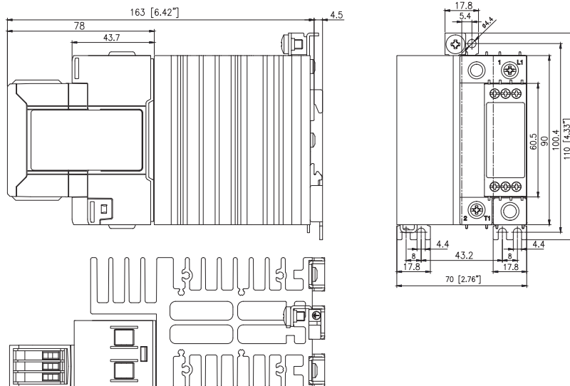
RGC1S60D90GGEP (extern zu liefernder Lüfter - keine Anschlüsse am RG-Modul)
