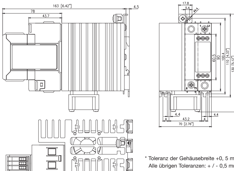
RGC1S60D90GGEP (extern zu liefernder Lüfter - keine Anschlüsse am RG-Modul)
