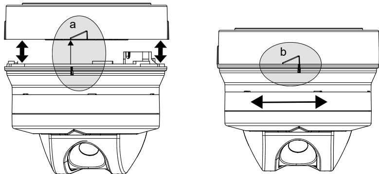
Fig. 6 Öffnen / Schließen
