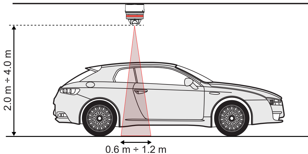
Fig. 2 Sensorhöhe und -abstand
