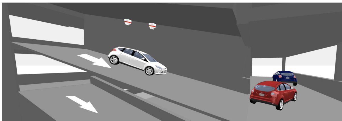
Die SBPSUSCNT-Sensoren funktionieren einwandfrei, wenn sie in der Mitte der Rampe platziert werden
