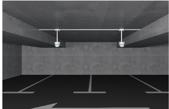
Positionieren Sie den SBPBASEA mindestens 5 cm unter dem Hindernis
