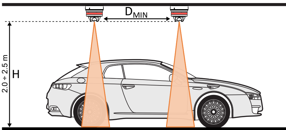
Fig. 3 Sensorhöhe
