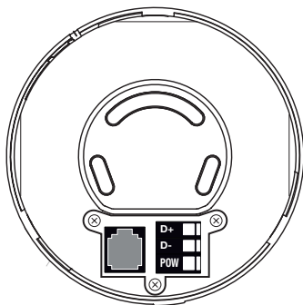
Fig. 5 Unterteil: an Decke montiert
