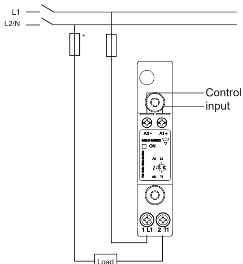
Variant uden over temperaturbeskyttelse
