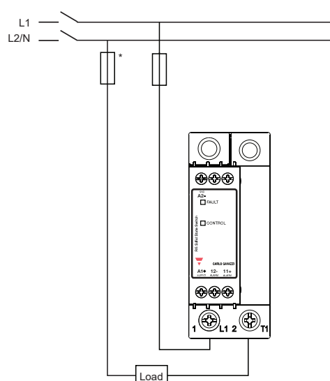
Variant med over temperaturbeskyttelse
