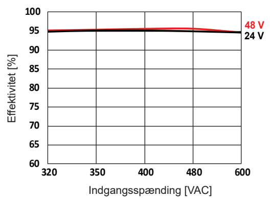
Effektivitet kontra indgangsspænding (fuld belastning)
