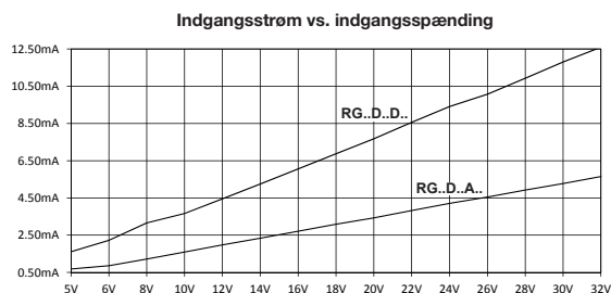
RG..D..D., RG..D..A..
