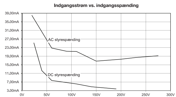
RG..A
