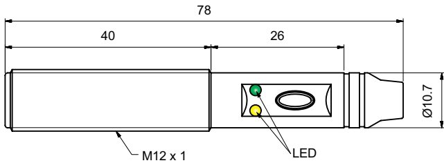
Fig. 6 Kabel CA18EAF...A2IO
