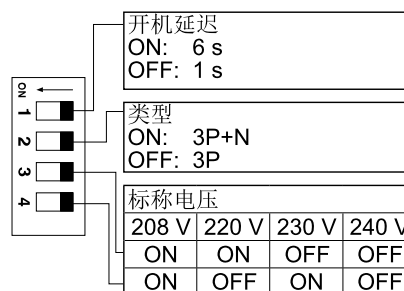
图 2DIP 开关设置表 (M23)
